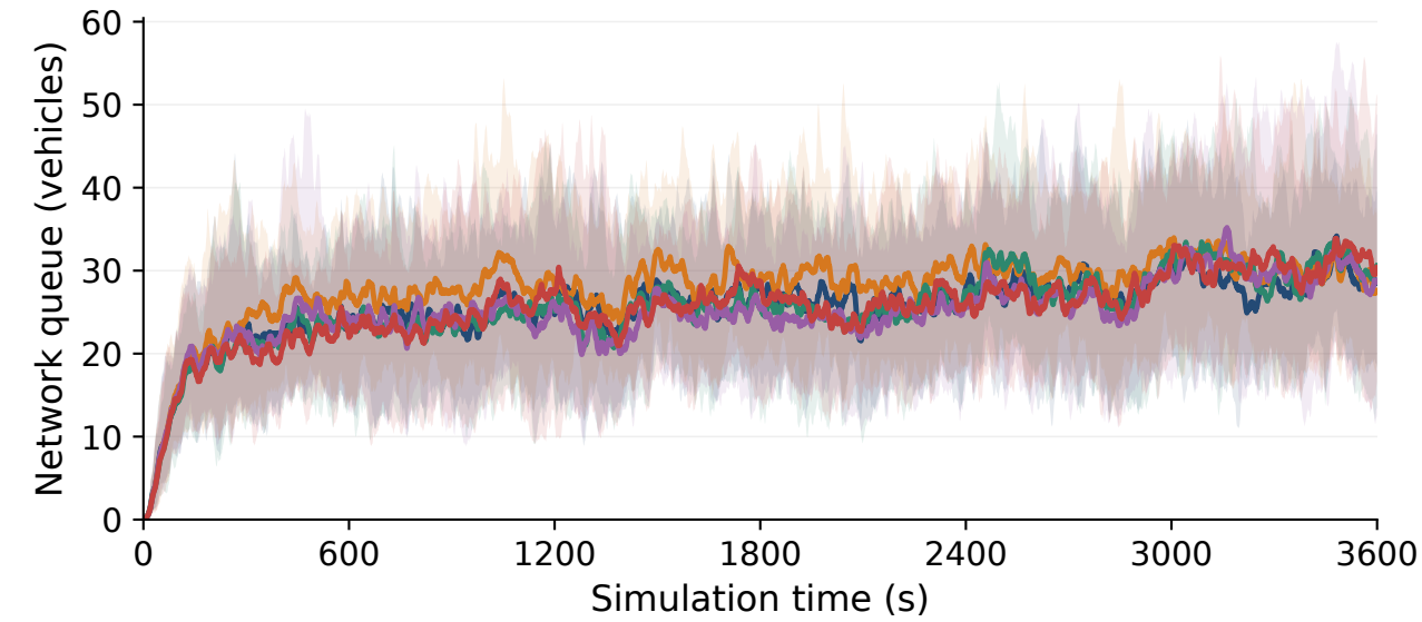
PPO
